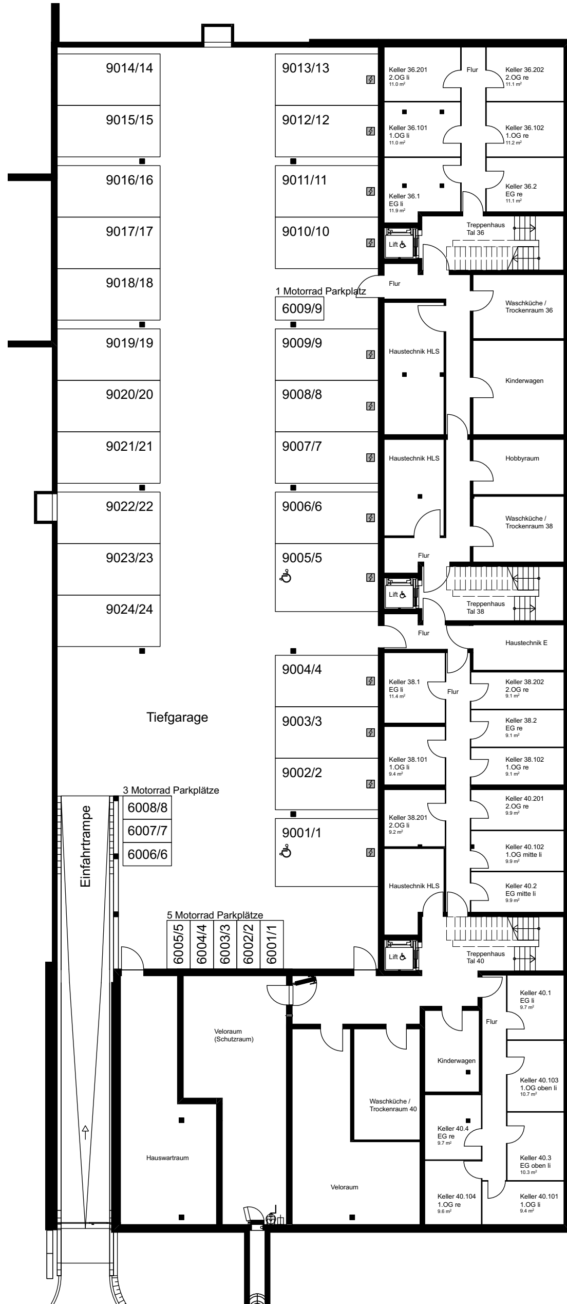
Untergeschoss
